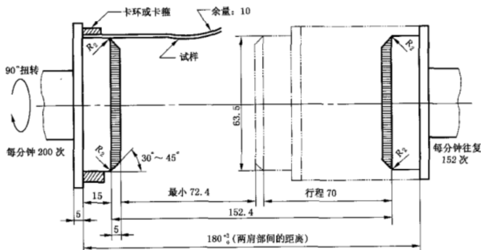
图 3 折皱屈挠设备示意图
