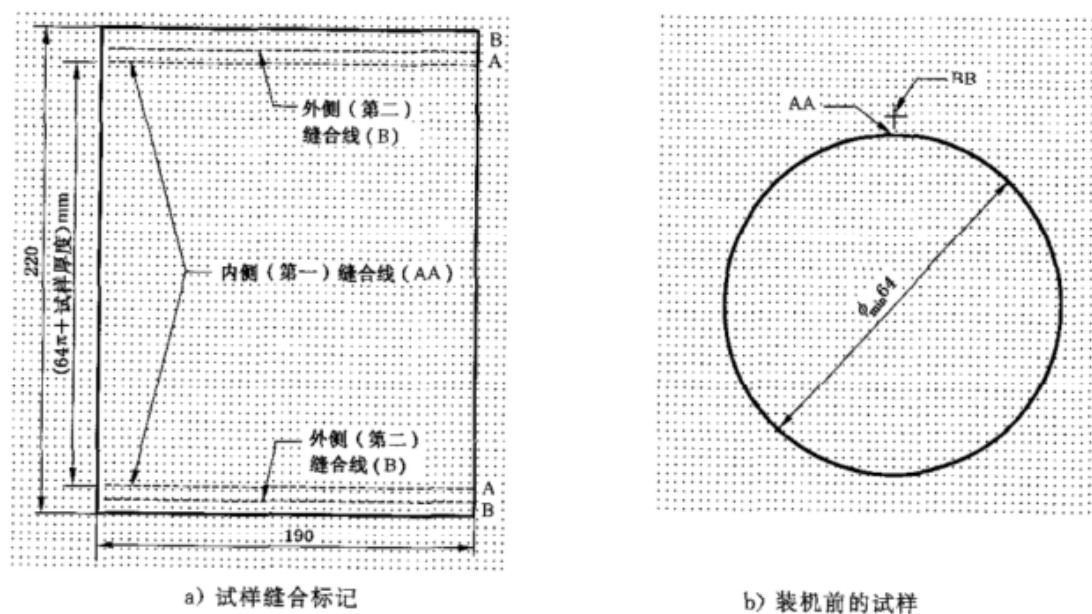
图4 折皱屈挠法用试样构形
