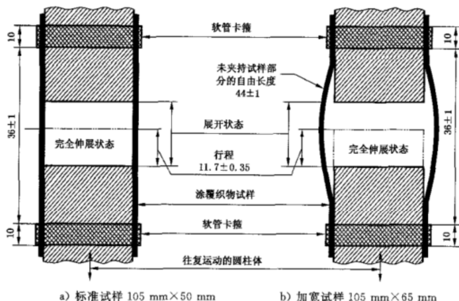
图2 试样安装
