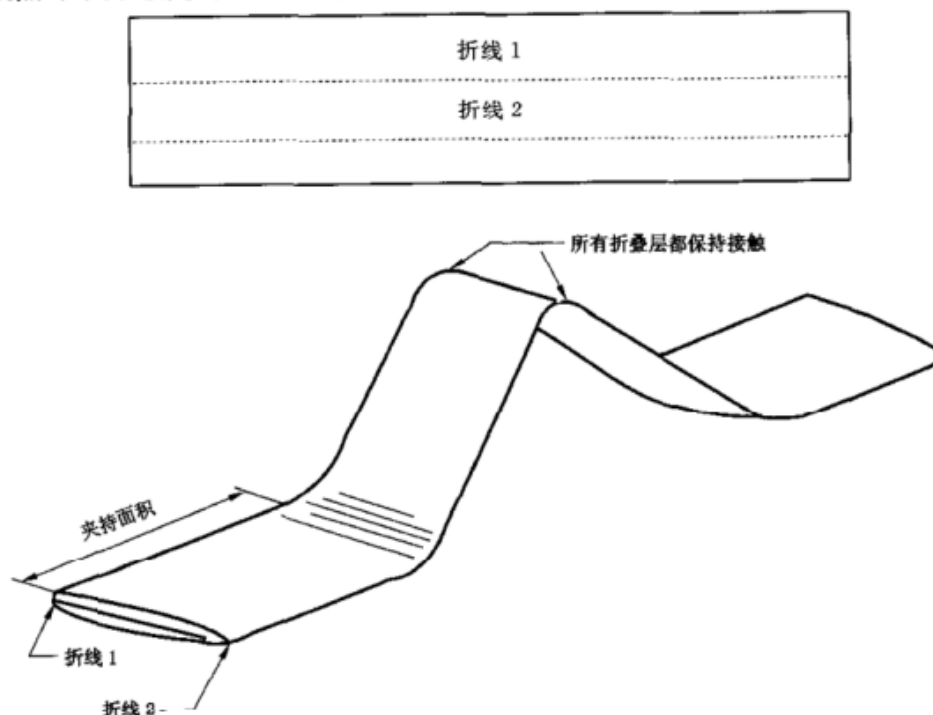
图 1 试样折叠和构形示意图
